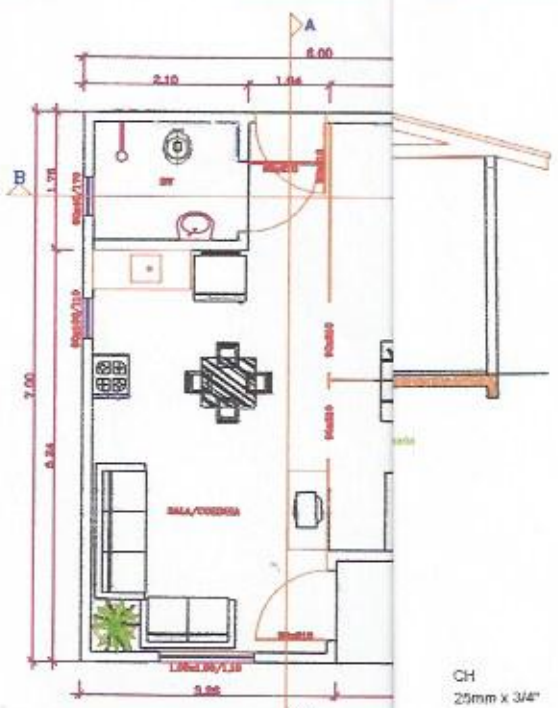
PLANTA BAIXA Área: 42,00 m 2
