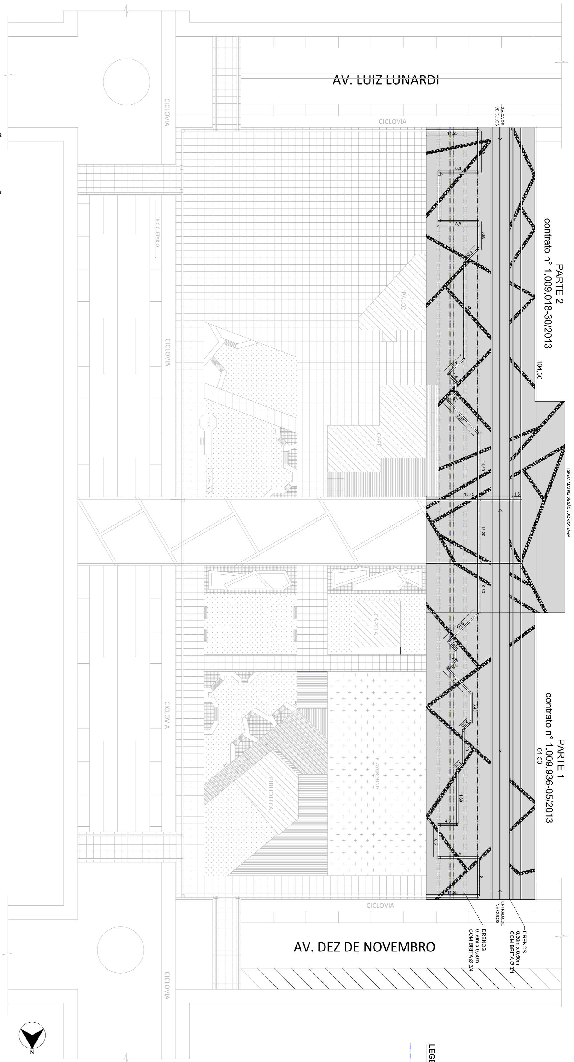
PLANTA DE PAVIMENTAÇÃO - CALÇADÃO ESC: 1/200
